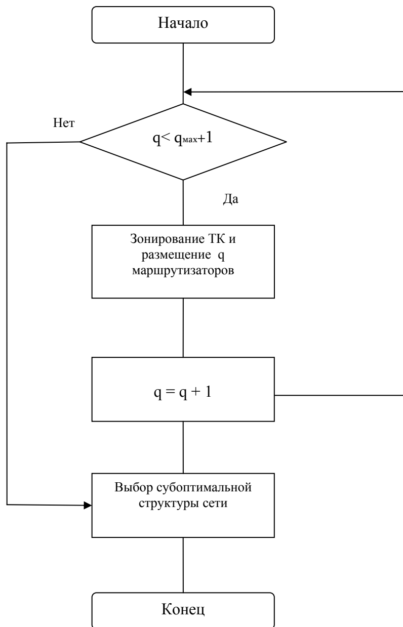
Рис. 4.4. Схема алгоритма размещения маршрутизатора
