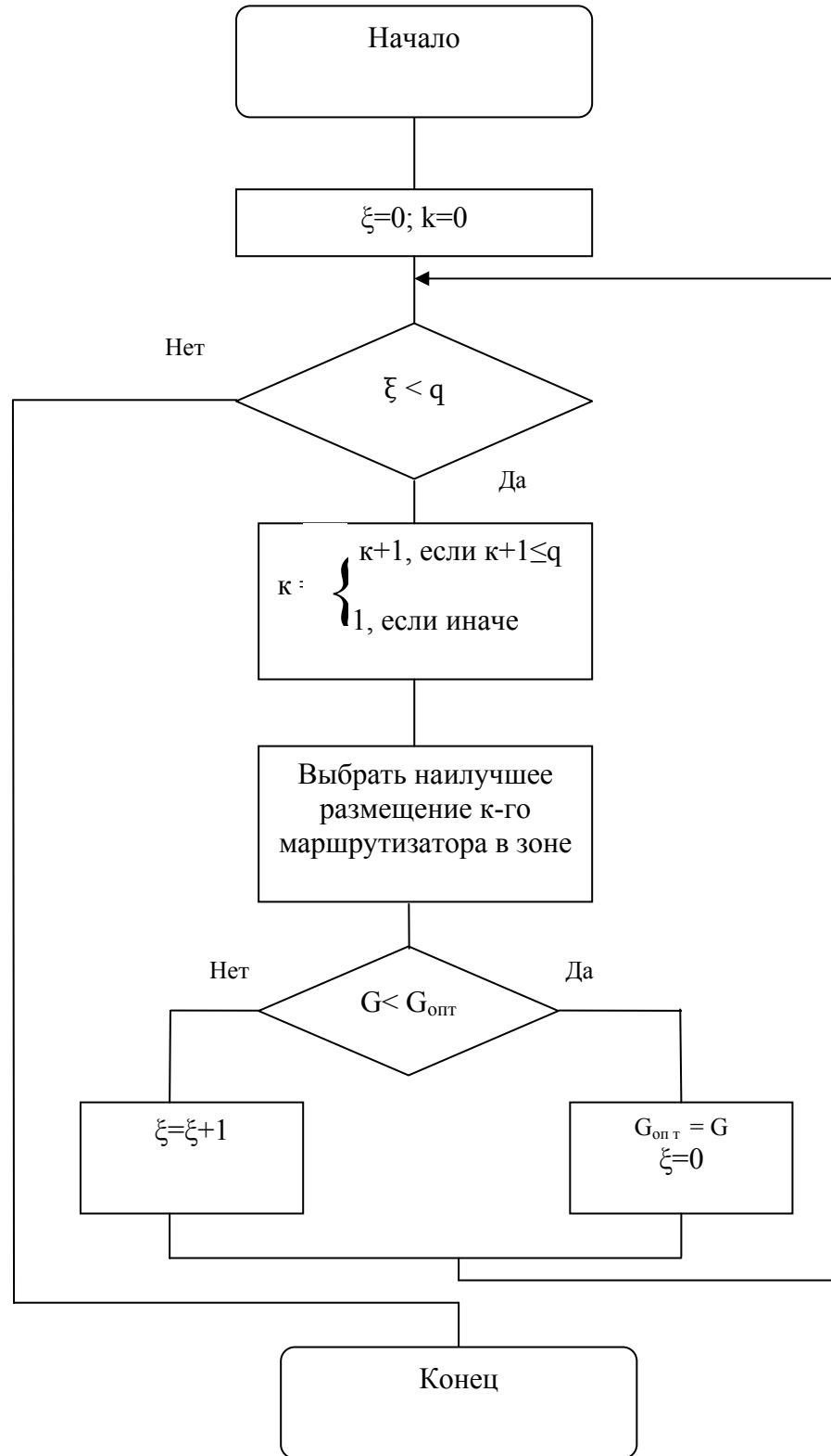
Рис. 4.6. Схема алгоритма выбора размещения q маршрутизаторов в фиксированных зонах
