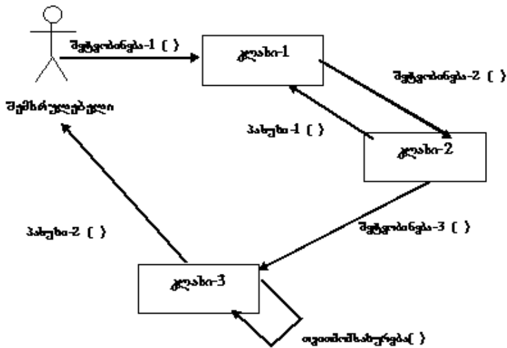
nax.3.8.2. Tanamoqmedebis diagrama
