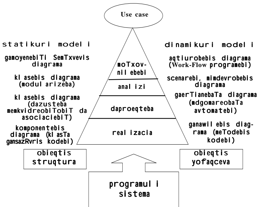
ნახ.3.1. პროგრამის სისტემის არჩევის განსაზღვრის ასპექტები UML-დიაგრამებით
