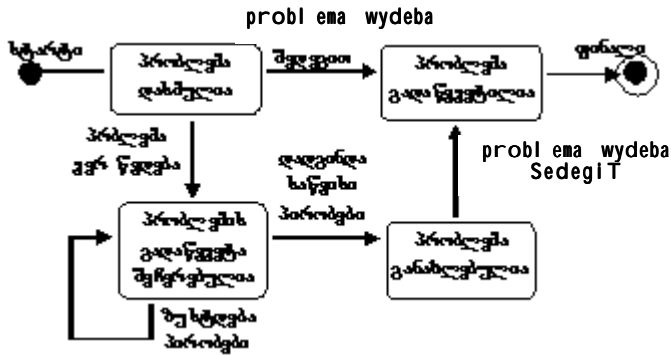
nax.3.10. mdgomareobaTa diagrama
