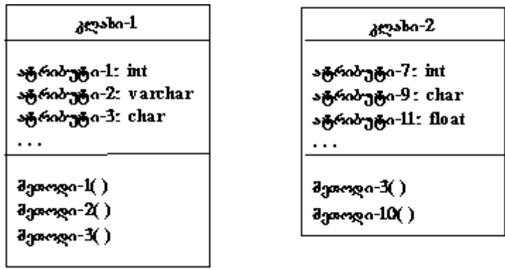
ნახ.3.7. კლასების დიაგრამა
